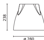
Opta diffuser 28
