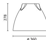
Opta diffuser 36
